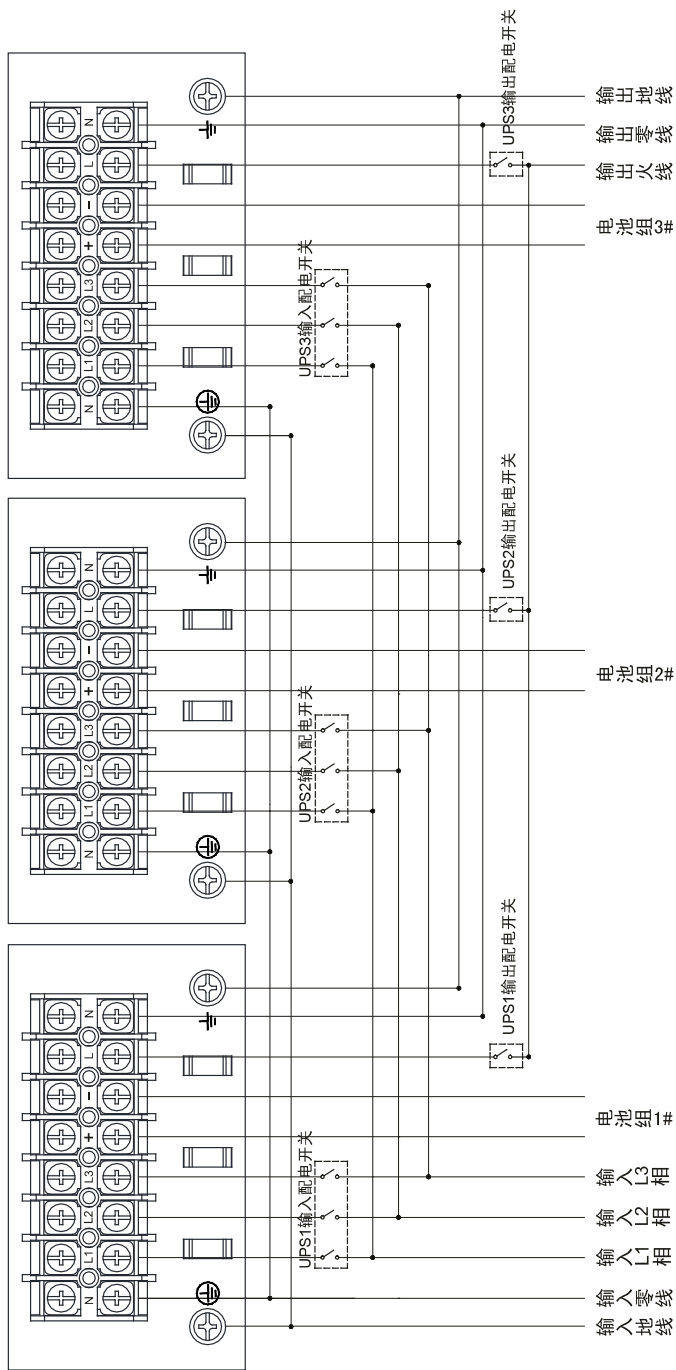
3C10KS并机接线图
