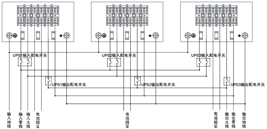
C6KS/C10KS并机接线图
