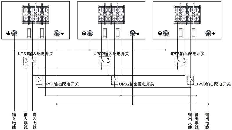
C6K/C10K并机接线图
